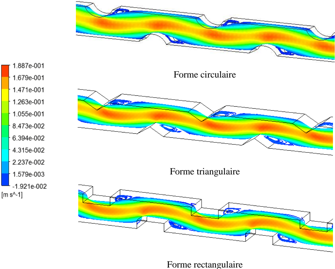
Figure IV.3 : Lignes de courant sur un plan horizontal (XY) pour Re = 20 , h/a = 0.3
