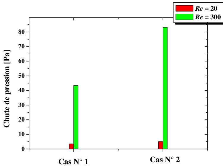
Figure IV.13 : Chute de pression en fonction du nombre des ondulations pour h/a = 0.3
