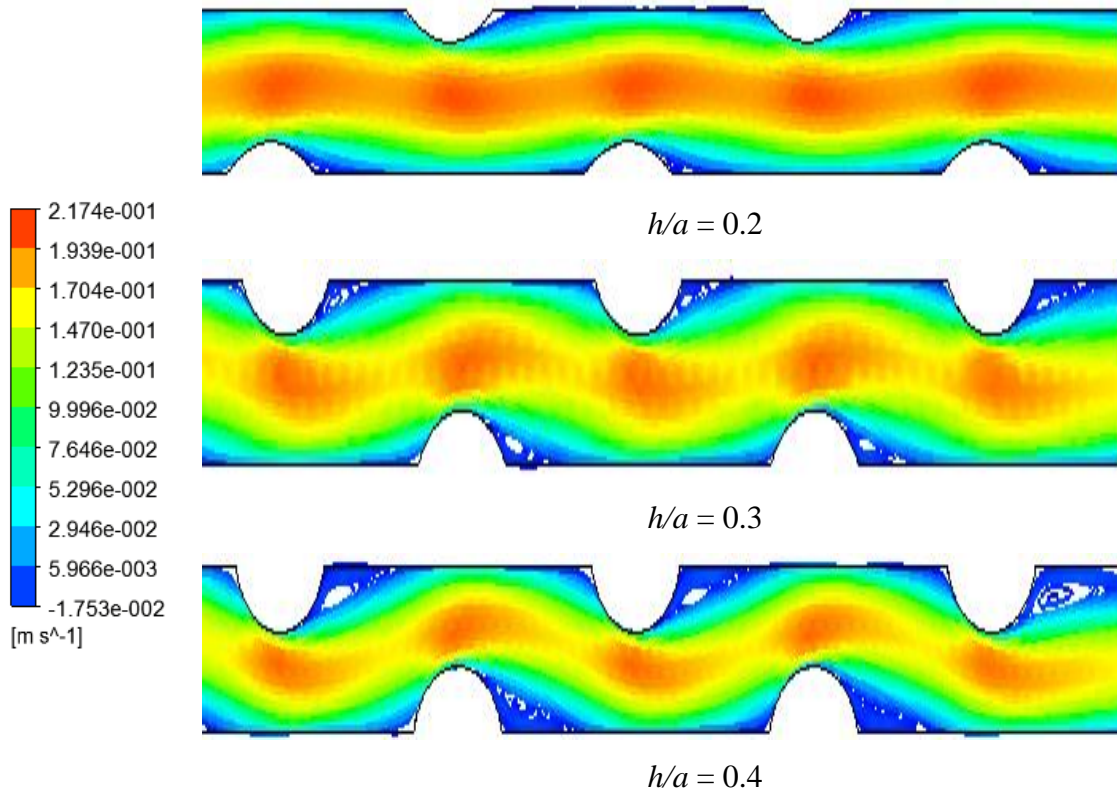
Figure IV.15 : Lignes de courant sur un plan horizontal ( XY ), pour Re = 20 , ondulation circulaire, Cas N° 1
