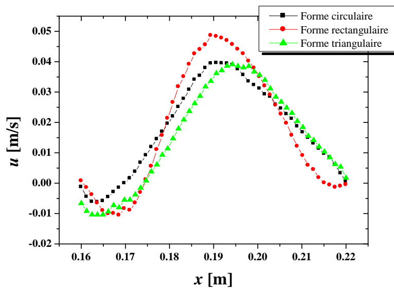
Figure IV.5 : Vitesse axiale en fonction du forme pour Re = 20 , h/a = 0.3 , z/a = 0.001
