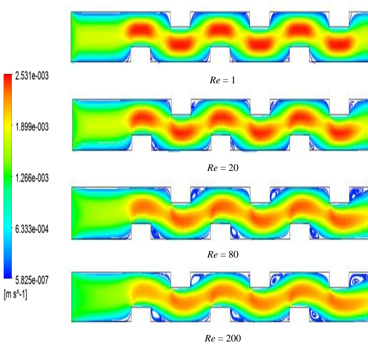
Figure IV.22 : Ligne de courant sur un plan horizontal ( XY ), pour h/a = 0.3 , ondulation rectangulaire
