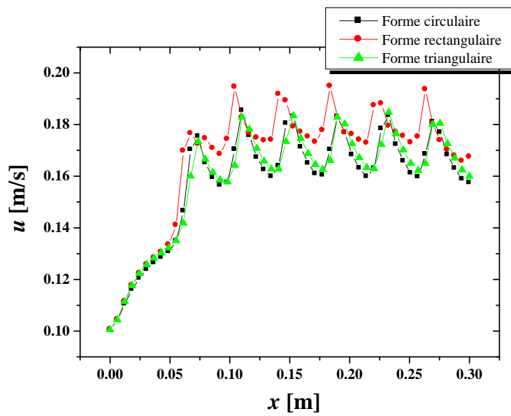
Figure IV.4 : Vitesse axiale en fonction du forme pour Re = 20 , h/a = 0.3 , z/a = 0.5
