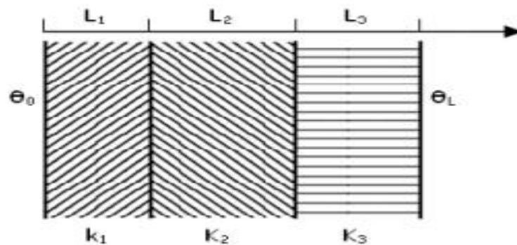
Figure I.5 : Schématisation du mur multicouche
